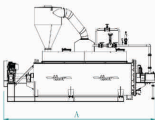
FILTRO ROTATIVO ÓLEO (Filtro Rotativo Aceite / Rotative Fat Drainer)
